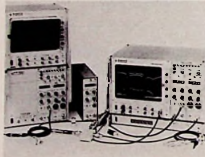
Polyskanner-Meßplatz von Knott Elektronik
