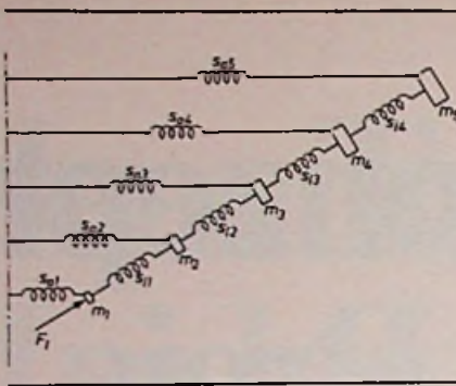
Bild 7. Darstellung eines Konus als System von Massen m und Federn mit Steifigkeiten s_l in longitudinaler Richtung und s_a in seitlicher Richtung. Von innen nach außen werden die Massen immer größer und die Federn s_a immer schwächer.
