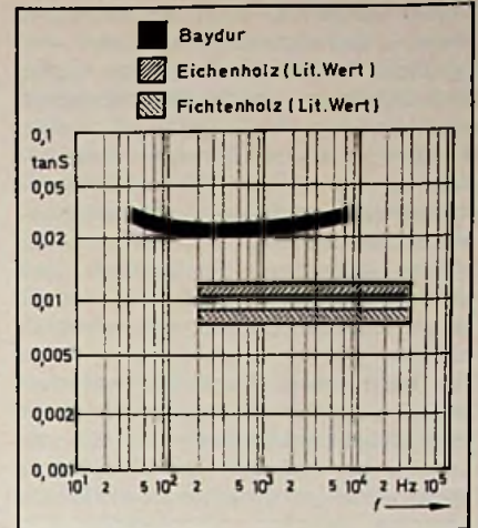
Bild 6. Akustisches Dämpfungsverhalten von Baydur
