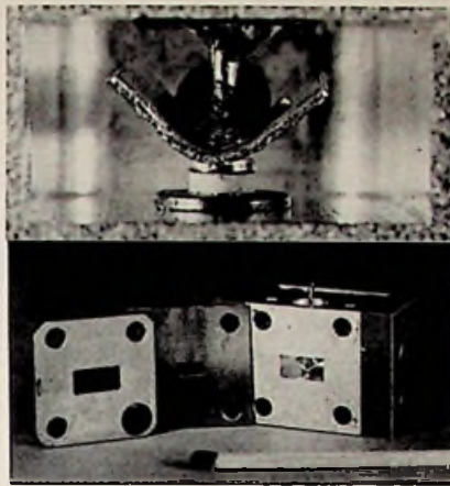
Bild 5. 35-GHz-Gunn-Oszillator, darüber eine Ausschnittvergrößerung
