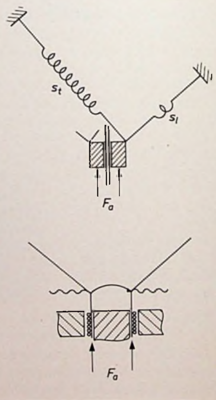
Bild 8. Darstellung der mechanischen Impedanz, die eine axiale Kraft F_a am Innenrand eines Konus erfährt. Diese Impedanz wird durch die gleichzeitige Wirkung zweier Federn dargestellt. s_l Impedanz für longitudinale Bewegungen. s_a Impedanz für transversale Bewegungen. Der Innenrand kann sich nur in axialer Richtung bewegen. Die longitudinale Impedanz ist in der Praxis am größten und ist maßgebend für die Ausschläge.
