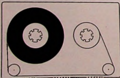
Bild 3. Prinzip der Zweiloch-Cassette für Links- und Rechtslauf
