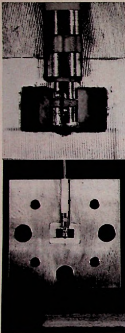
Bild 7. 86-GHz-Mischer, darüber eine Ausschnittvergrößerung
