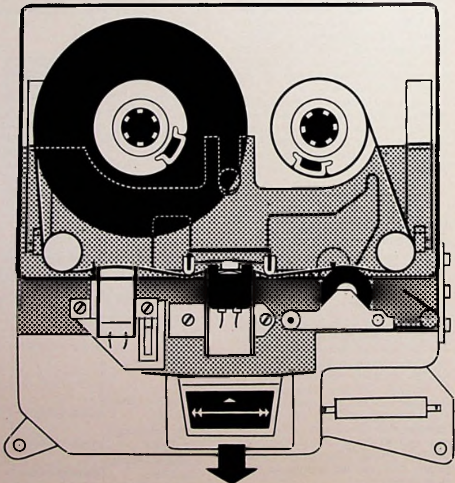
Bild 4. Antriebssystem und Kopfträgerplatte beim Cassetten-Recorder
