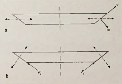
Bild 6. Schwingungsform eines konischen Rings bei Resonanz (a) und Antiresonanz (b). u longitudinale und w transversale Verschiebung. Bei der Antiresonanz ist trotz des Antriebs durch eine longitudinale Kraft F_l die longitudinale Verschiebung gleich Null.
