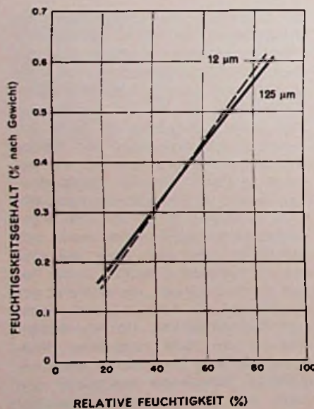
Bild 8. Einfluß der relativen Luftfeuchte auf die Aufnahme von Feuchtigkeit bei der Mylarfolie
